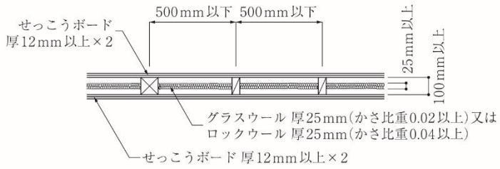
(A) 平面図
