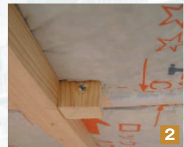
2 吊木周りに隙間を生じさせないようにマットを突き付けます。
