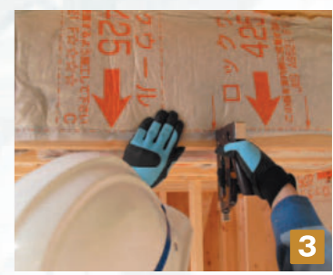
3 下がり壁部分に、寸法に合わせてカットしたマットを充填していきます。
