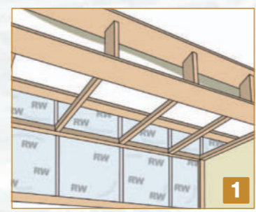
1 外壁を先行して充填し、その後下がり壁と野縁を施工します。
